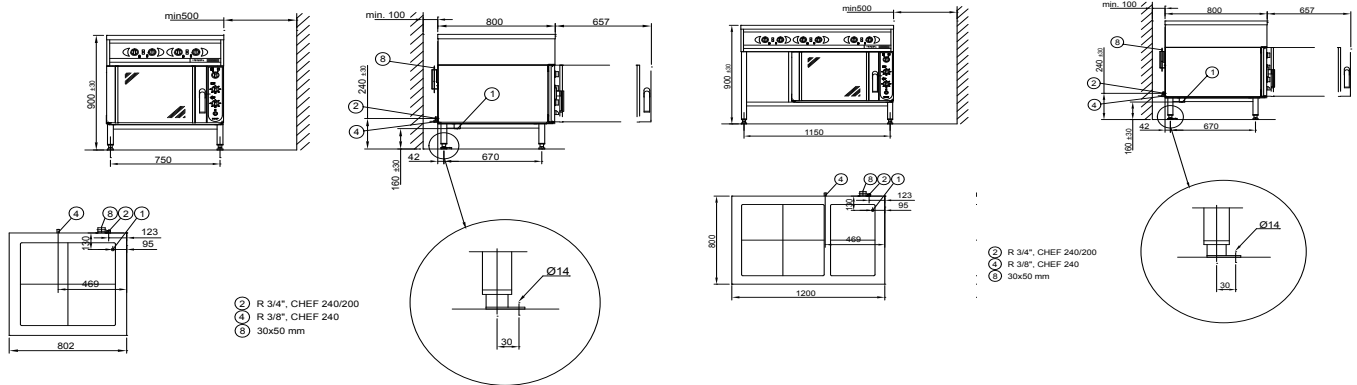
Futura RP4 four chef 22 code 3751993
