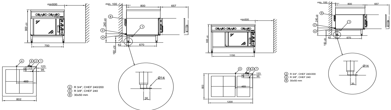
Futura RP4 four chef 24 code 3751997
