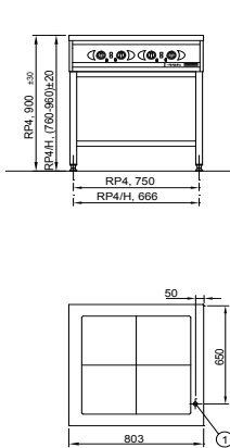
Futura RP4 code 3494358
